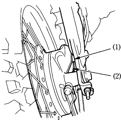
(2) Slot
